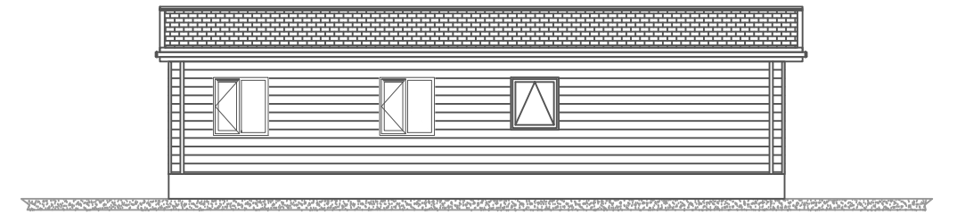
Elevation B
