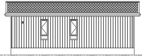
Elevation B
