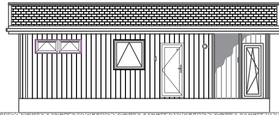
Elevation A
