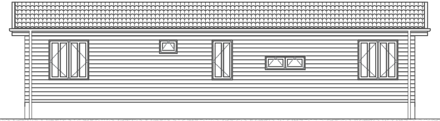
B Elevation
