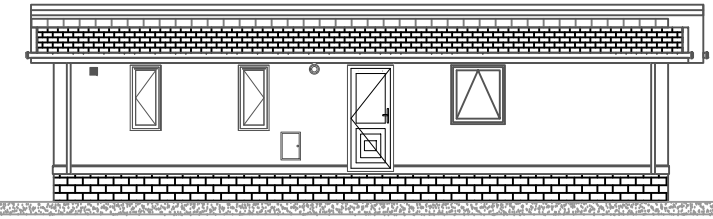
Elevation B
