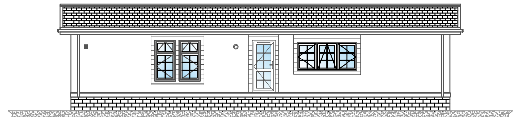
Elevation B
